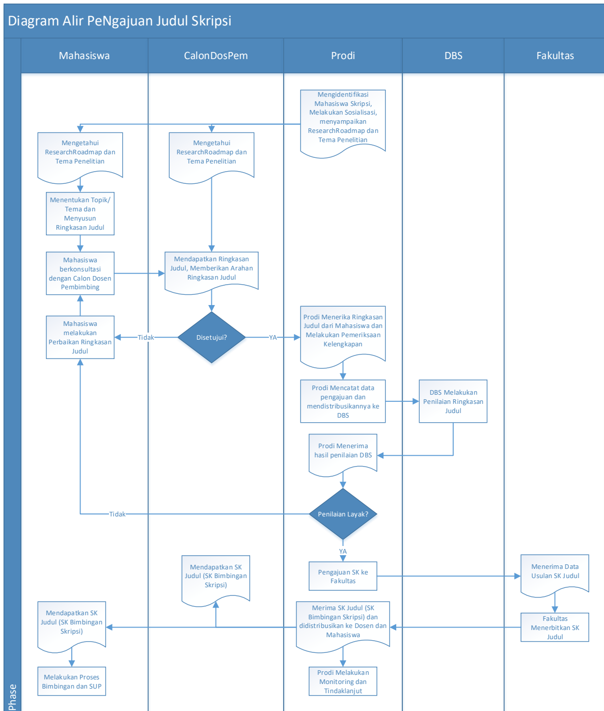
Gambar 1. Flowmap Pengajuan Judul Skripsi
